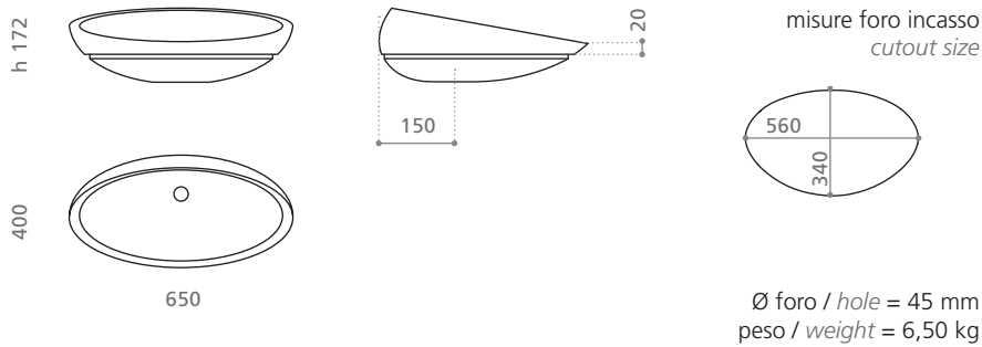
Kool XL FL
