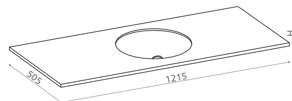
Bolla sotto 1215 TOPG121
