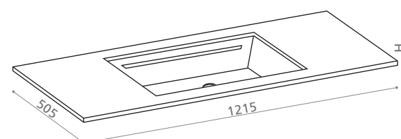
Yacht sotto 1215 TOPG121
